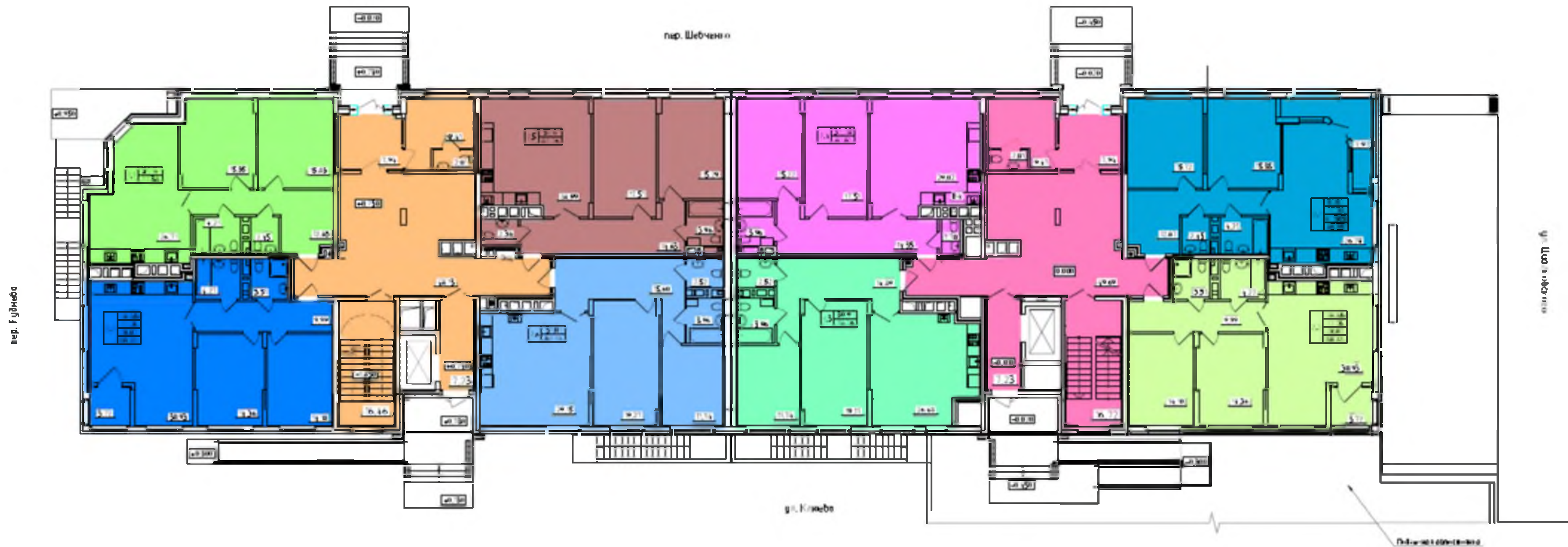
План на отн. 1 этажа на отн. 0,000, +0,750
